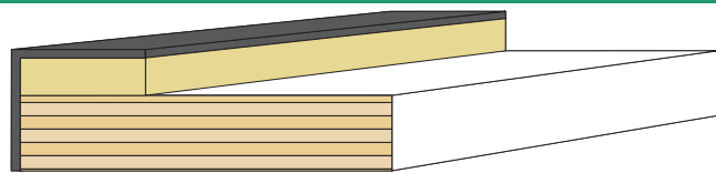
Multiplex WBP 60 mu gegronde met opdiklat en PVC-hoeklijn
