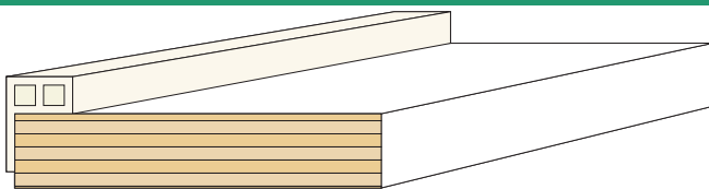
Multiplex WBP 60 mu gegronde met kunststof opdikprofiel Als alternatief voor opdiklat met PVC-hoeklijn
